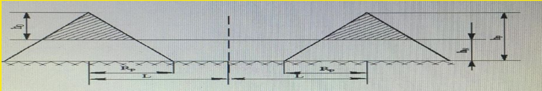
Сурет 2 – Үйіндіге техникалық рекультивациялауда топырақгрунттарын төгу сұлбасы
